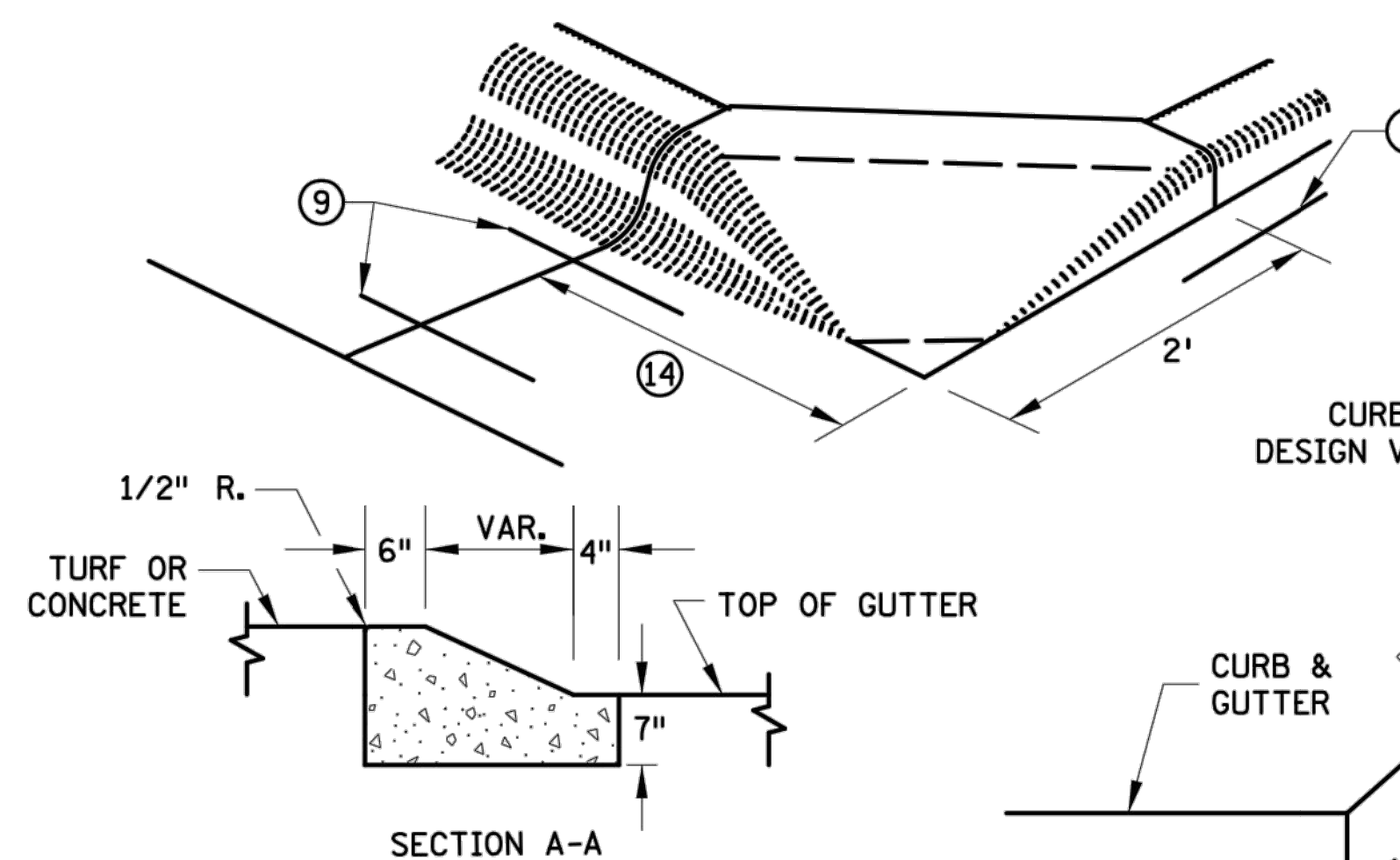
SECTION A-A
