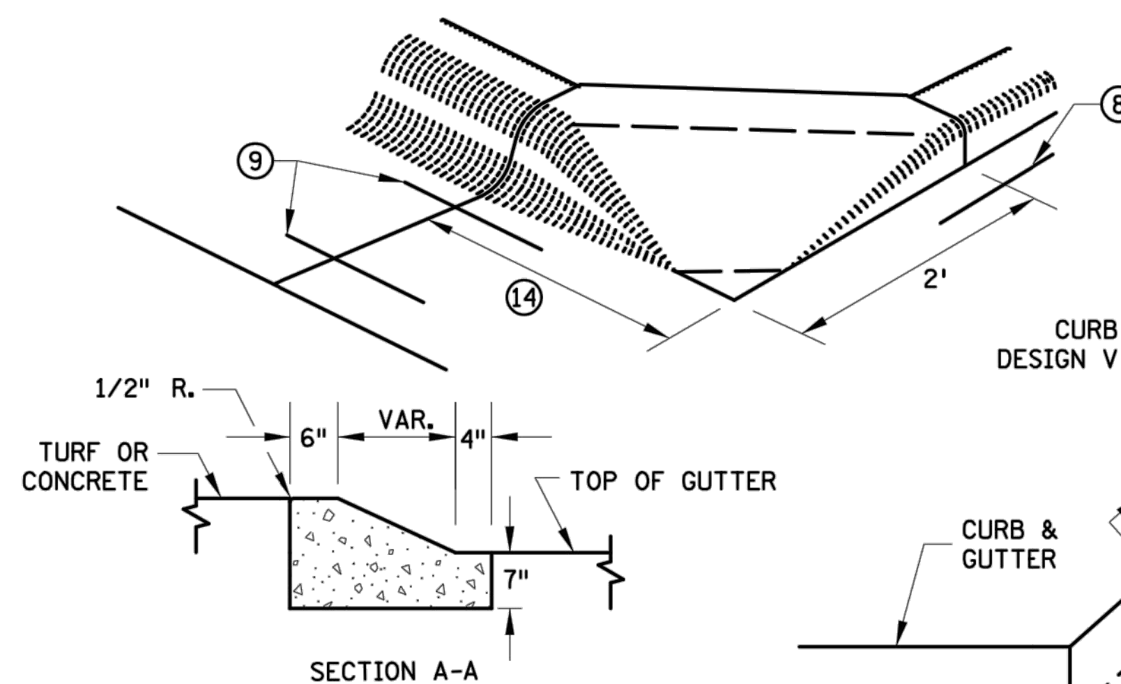
SECTION A-A
